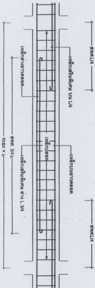
ขยายหน้าตัดคาน(ด้านยาว)
