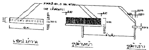
แบบขยายไม้กวาดลากผิวพื้น ค.ร.ล.
