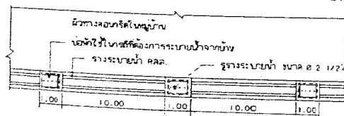
แปลนร่างระบายน้ำ คลล.ในหมู่บ้าน
