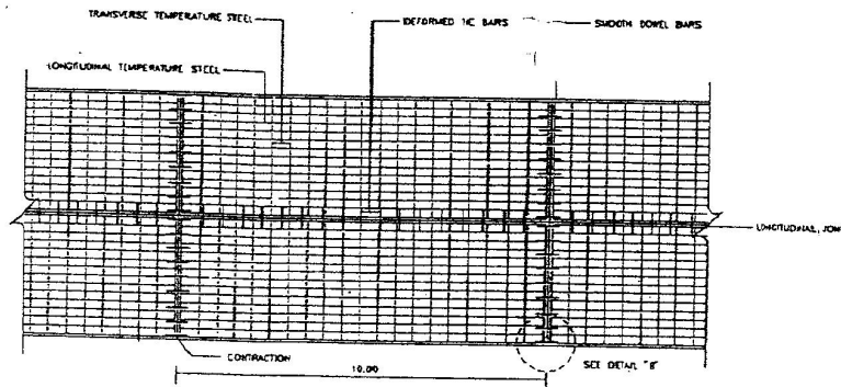
แบบแผนและการเสริมเหล็กถนน ค.ร.ล.
